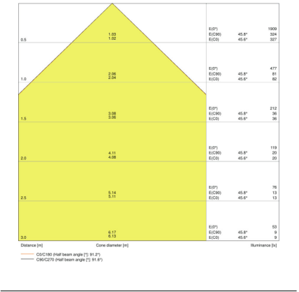
FL PFM 10 W 3000 K SYM 100 WT
