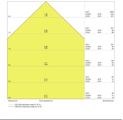
FL PFM 10 W 4000 K SYM 100 BK
