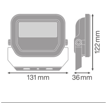
FL PFM 10 W 3000 K SYM 100 BK, FL PFM 10 W 3000 K SYM 100 WT, FL PFM 10 W 4000 K SYM 100 BK, FL PFM 10 W 4000 K SYM 100 WT, FL PFM 10 W 6500 K SYM 100 BK, FL PFM 10 W 6500 K SYM 100 WT
