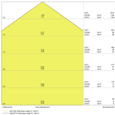
DP 1200 18W 865 IP65 GY
