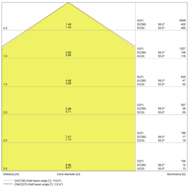
DP 1500 26W 865 IP65 GY
