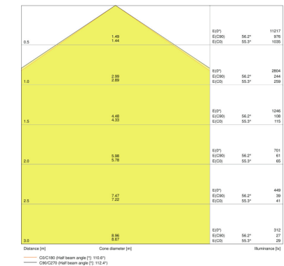
DP 1500 58W 840 IP65 GY
