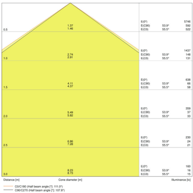
DP 1200 32W 830 IP65 GY
